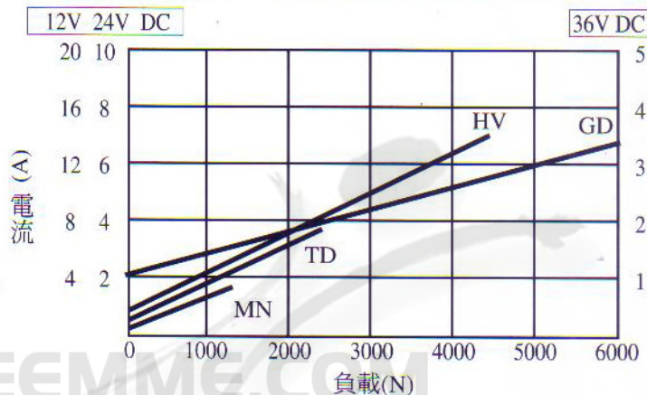
電流與負載關係圖
