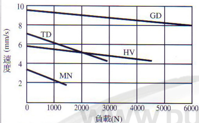
速度與負載關係圖
